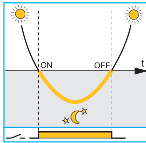
Typ 11.41 "Null-Hysteresis-Prinzip" beim Dämmerungsschalter
