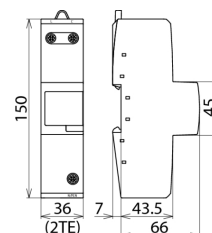
Maßbild DBM 1 440
