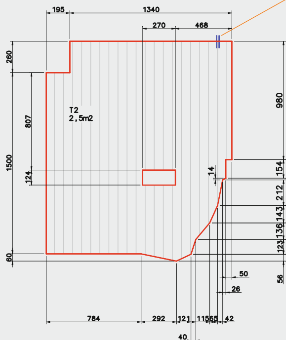
Beispiel für Netzheizmatten auf Maß
