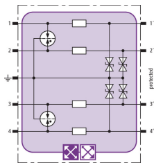
Prinzipschaltbild BXT ML4 BE 12
