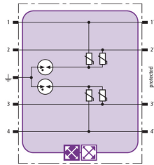
Prinzipschaltbild BXT ML4 MY 250
