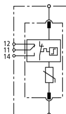
Principalschaltbild DG S 320 FM
