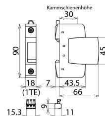
Maßbild DG S 320 FM
