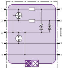
Prinzipschaltbild BXT ML2 BE S 5
