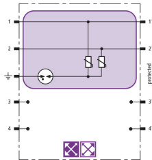
Prinzipschaltbild BXT ML2 MY 250
