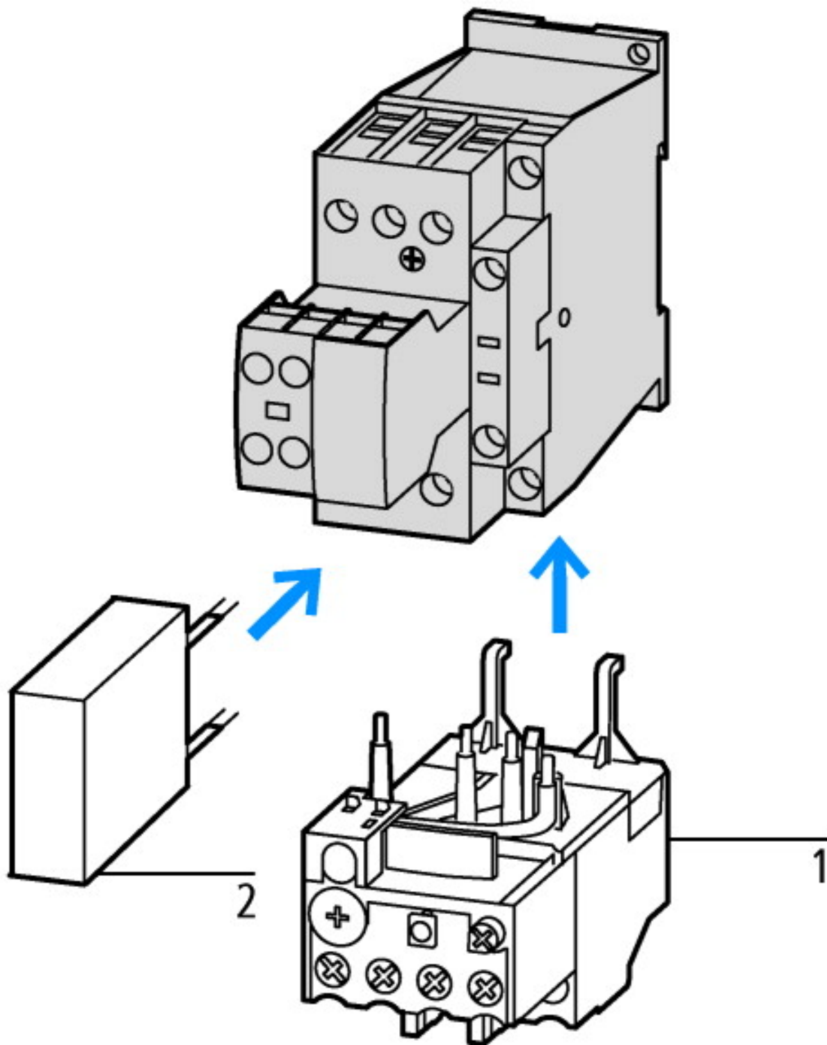
1: Motorschutzrelais 2: Schutzbeschaltung
