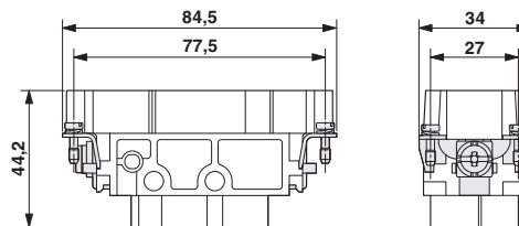
Buchseneinsatz
