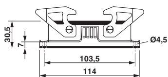
Maßzeichnung
