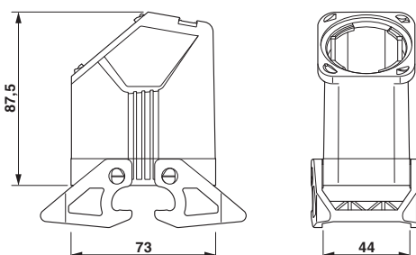
Maßzeichnung
