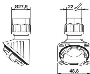
Maßzeichnung
