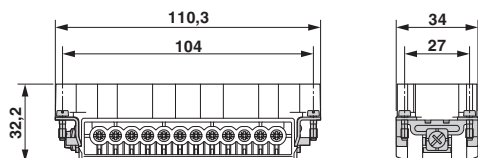
Maßzeichnung
