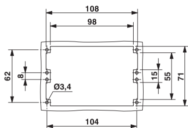
Montageausschnitt bei Verwendung ohne Gehäuse
