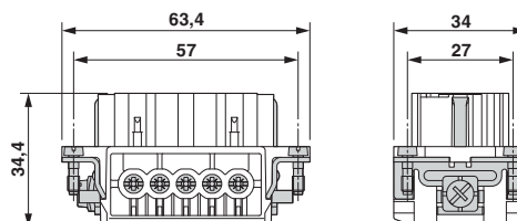
Maßzeichnung
