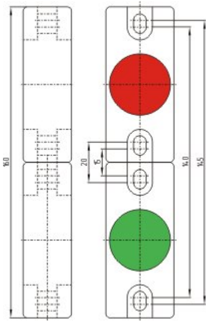
Maßzeichnung (Sonstige)
