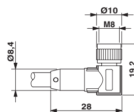
Buchse M8 x 1, gewinkelt, geschirmt
