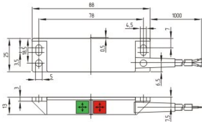
Maßzeichnung (Grundgerät)
