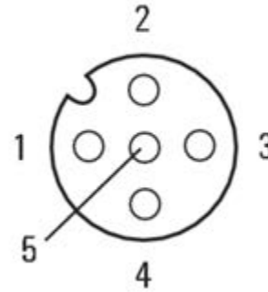
Buchse
