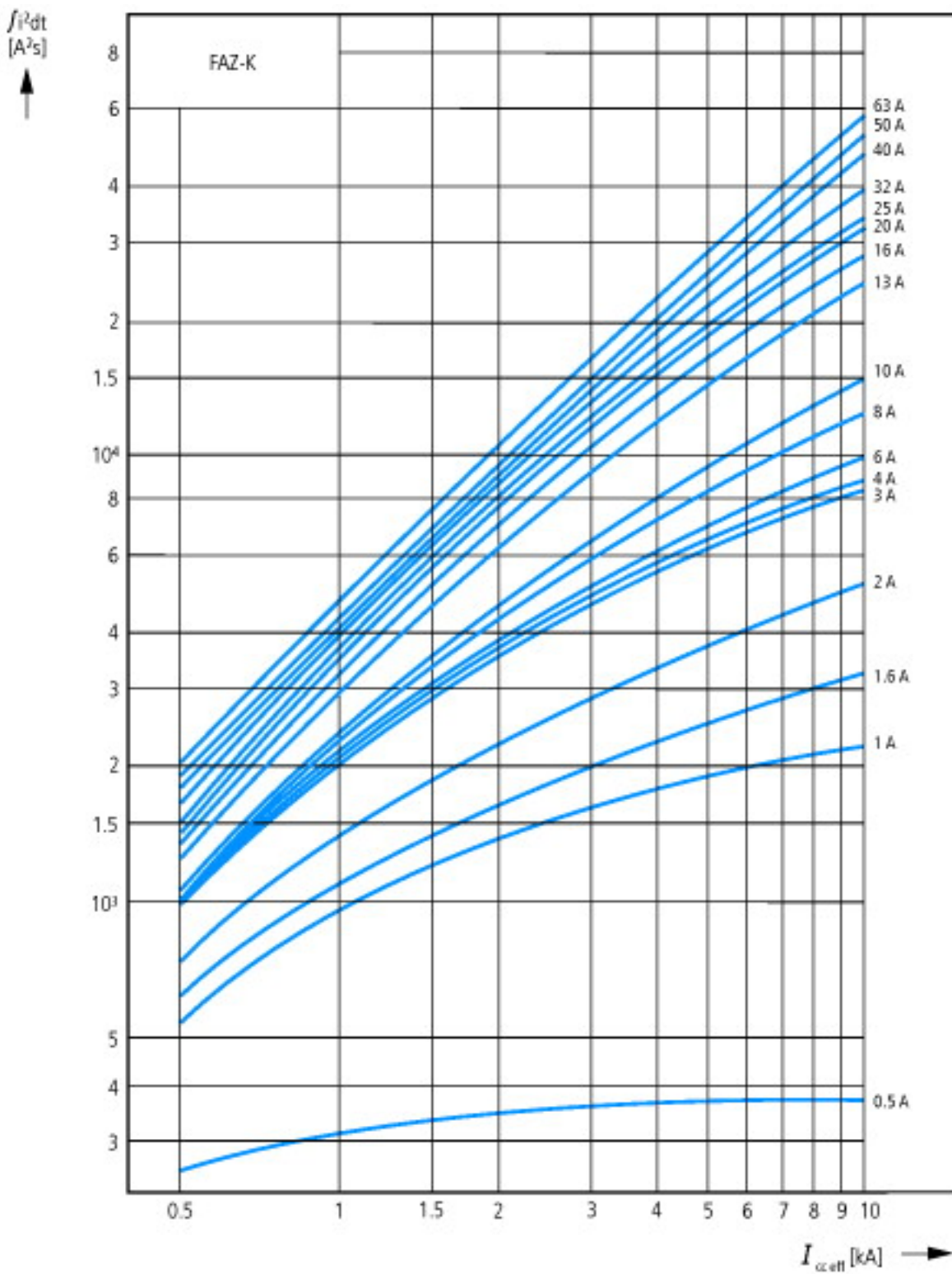
Durchlassstrom I_D Ermittlung nach IEC/EN 60898
