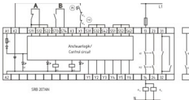
Schaltungsbeispiel
