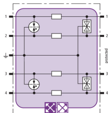
Prinzipschaltbild BXT ML4 BE HF 5
