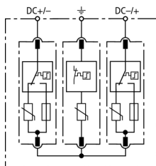
Prinzipialschaltbild DG M YPV SCI 1000
