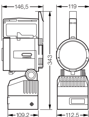
SEB 8 DIN/SEB 8 L DIN
