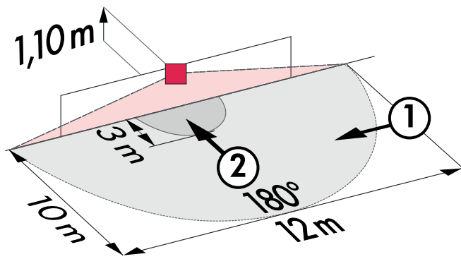
Reichweitendiagramm
