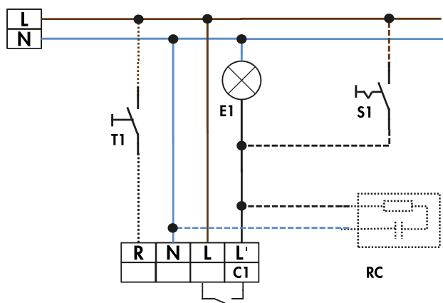
Schaltbild
