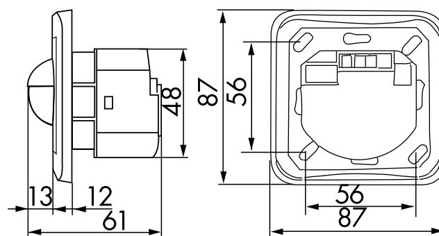
Bemaßung
