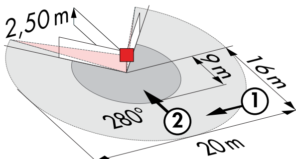
Reichweitendiagramm
