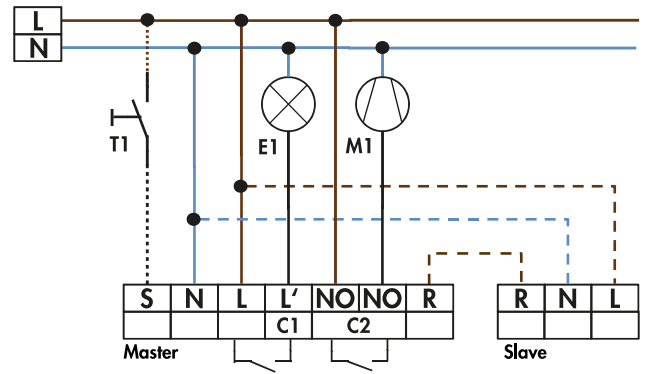
Schaltbild
