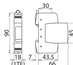
Maßbild DR M 2P 255
