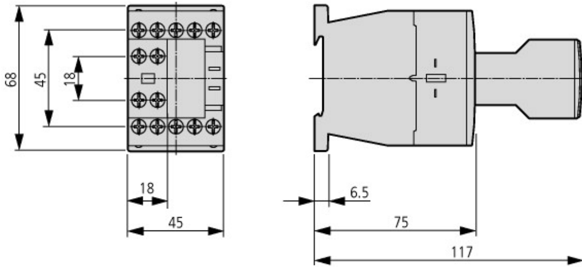
Schütze mit Hilfsschalterbaustein
