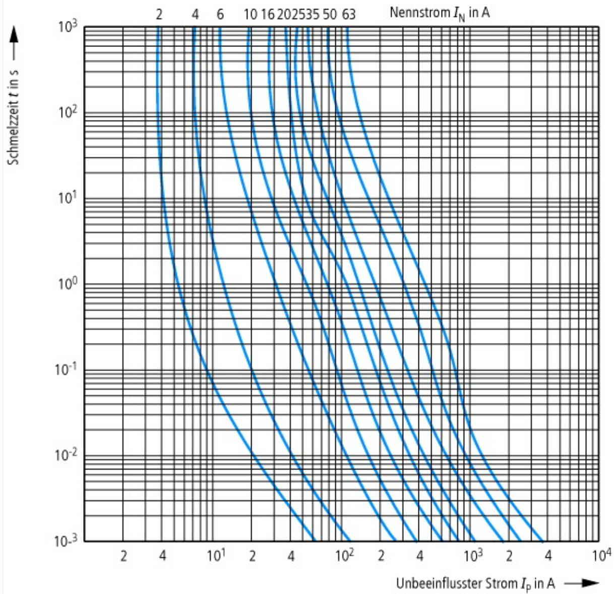
Zeit-Stromkennlinie D0-Schmelzeinsätze 2...63 A gG(L)
