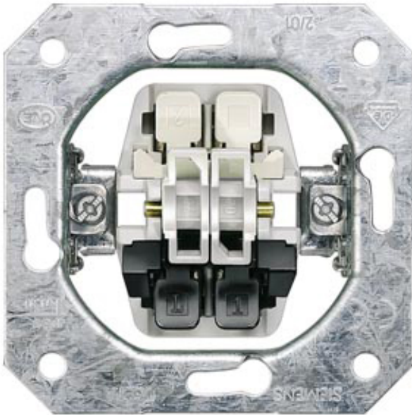
DELTA SCHALTER-GERÄTEEINSATZ UP, JALOUSIESCHALTER 16A 250V MECHANISCH VERRIEGELT
