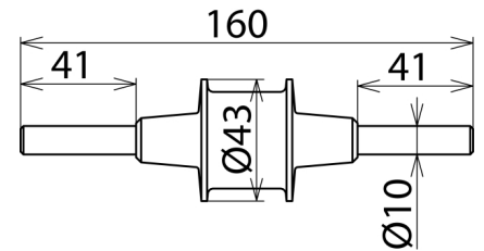
Maßbild KFSU
